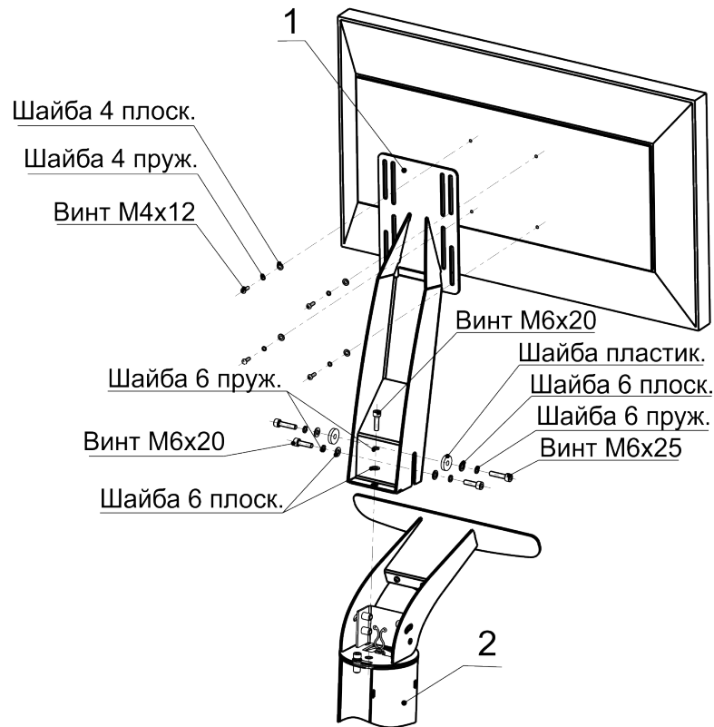
Рисунок 4.7 - Установка монитора
