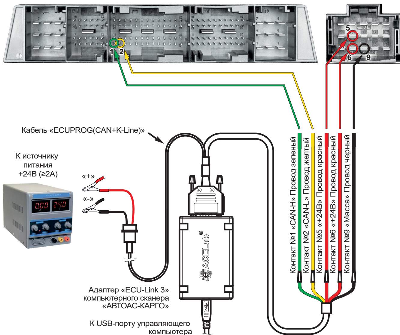
Рис. Схема подключения.
